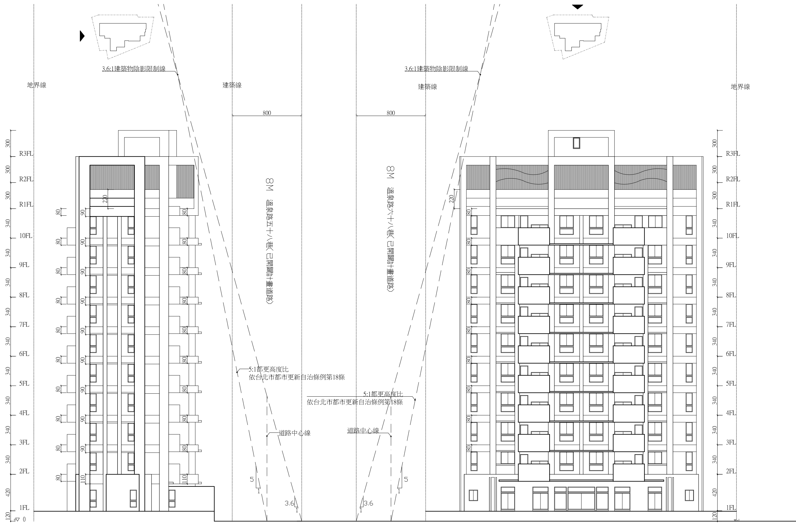
西向立面圖 S=1/250
